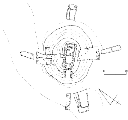
図3 たぬき塚古墳墳丘平面図
